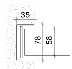
Einlauf V3 Variante Volltürblatt
