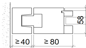
Einlauf V2 Variante Glas 1x Schutzglas flächenbündig
