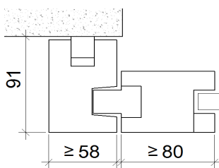
Einlauf V1 Variante Glasrahmen
