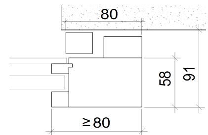
Hinten H1 Variante Glas 1x Schutzglas flächenbündig
