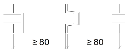
Mitte Mi1 Variante Glasrahmen
