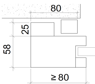
Hinten H1 Variante Glasrahmen
